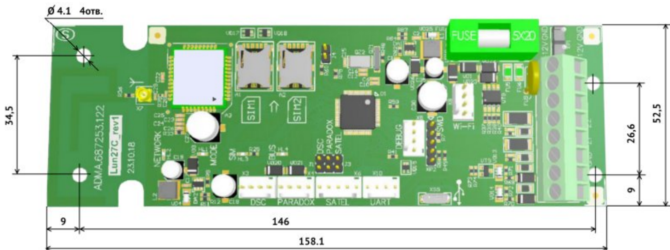
Рисунок 3. Габаритные и присоединительные размеры платы УСО
